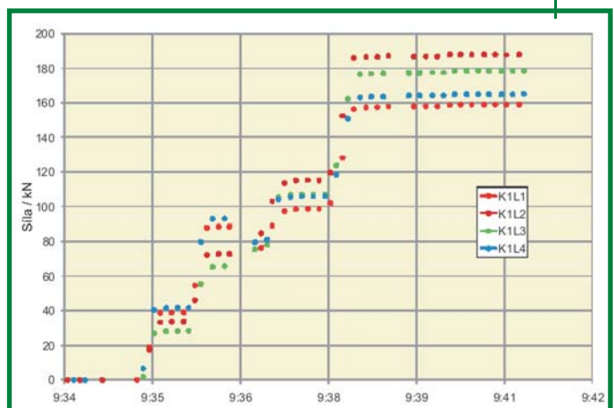
graf kontroly napínacího procesu zemní kotvy
